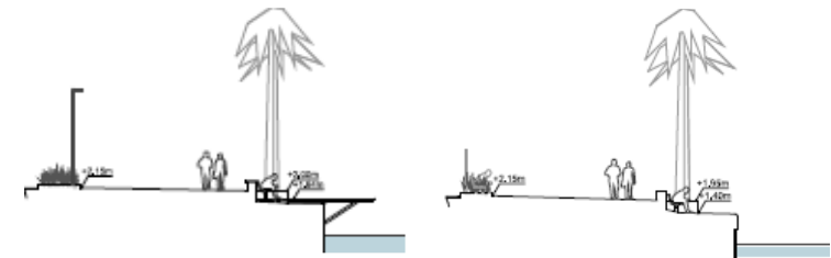
Secciones Tipo Muelles 1 y 2.
