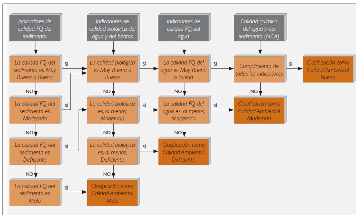
Figura 3. Proceso de integración jerárquica de los elementos de calidad (ROM 5.1-13:Fig 6.2).
