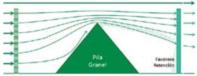
Las pantallas porosas a barlovento y sotavento evitan la salida de polvo.
