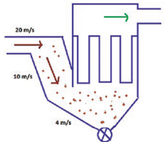
Prefiltrado mediante cámara de decantación.
