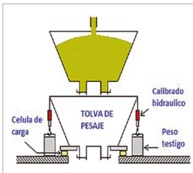
Esquema de cargador con dosificador de carga
