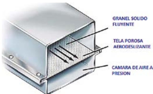
Esquema de transportador de lecho
